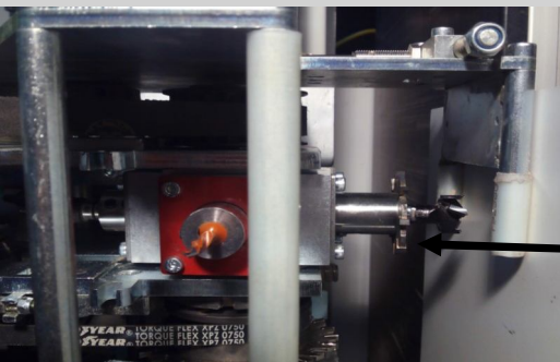
Taladro N°3. Broca de 20mm para Taladros frontales minifix * OPCIONAL : Pack Fresado Sierra ranurar cantos
