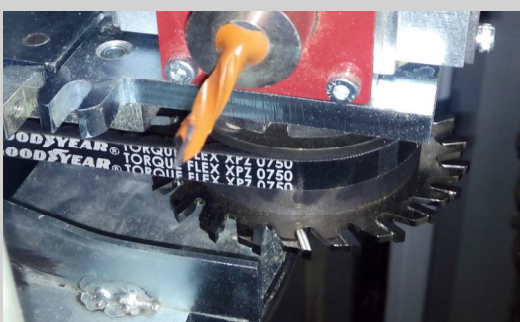
Portaherramientas N°5. Sierra para ranurar fondo
