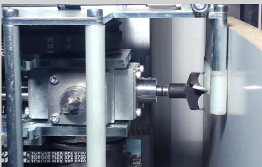
Taladro N°4. Broca de 35mm para Taladros frontales de Bisagra
