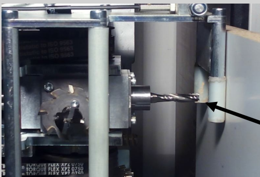
Taladro N°2. Broca de 8mm para Taladros frontales y de canto. * OPCIONAL : Pack Fresado Fresa 8 mm para taladros frontales, de canto y fresados auxiliares.
