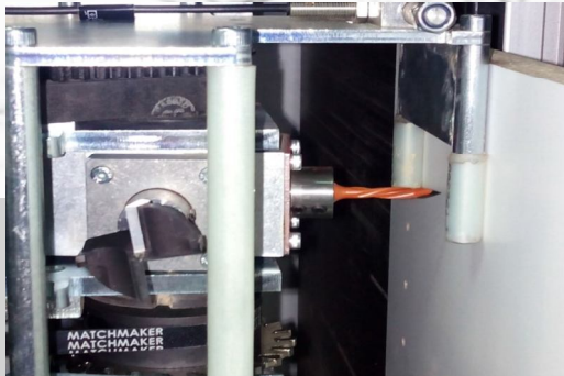
Taladro N°1. Broca de 5mm para Taladros frontales y de canto.
